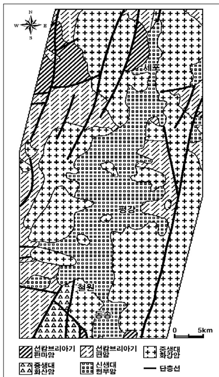
그림 2. 연구 지역의 지질
