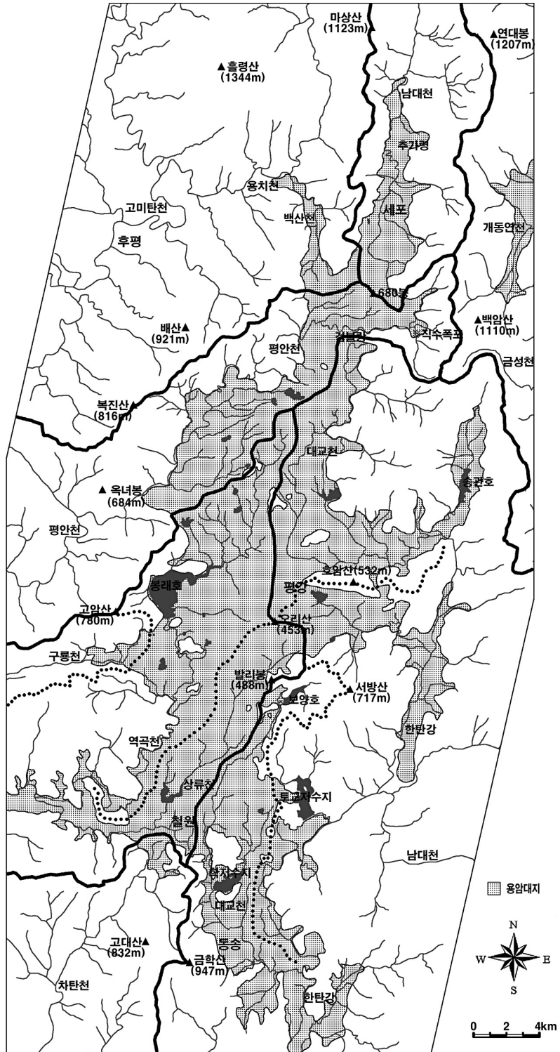
그림 7. 철원-평강 용암대지와 하계망
