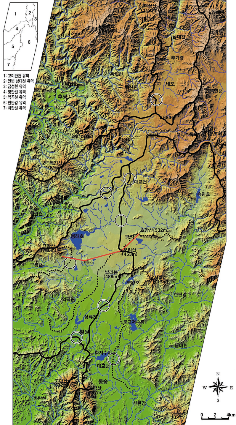
그림 6. 철원-평강 지역의 지형
